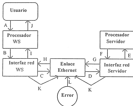
Figura 2.1.2- Entidades y Eventos de un sistema LAN
