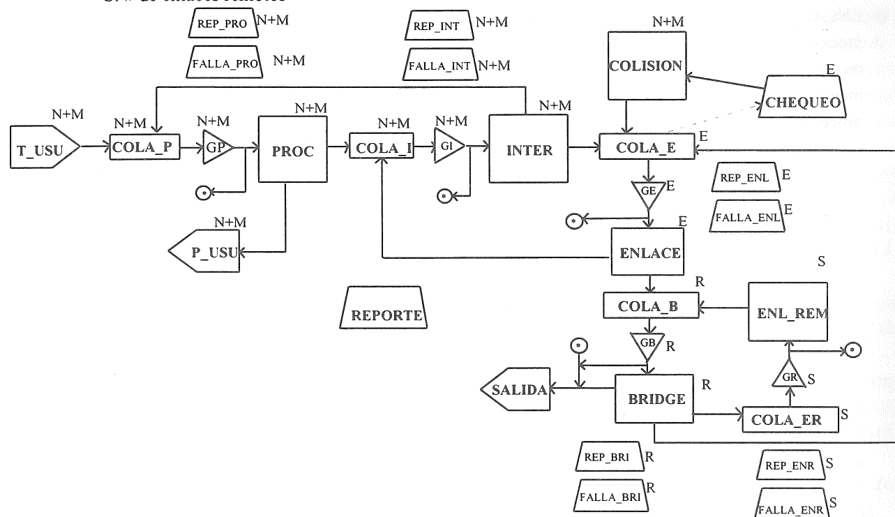
A continuación se describen funcionalmente los nodos que conforman el modelo Glider genérico de una LAN.
