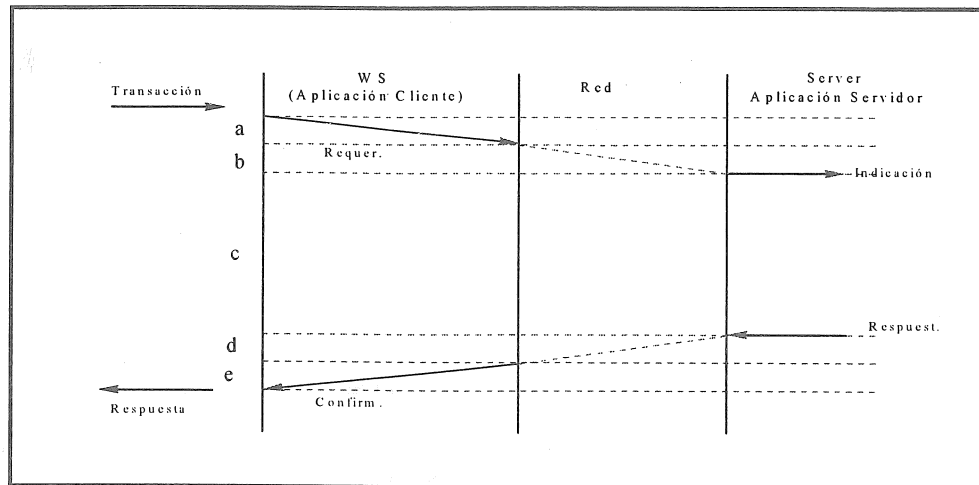
Figura 2.1.1. Comunicación entre dos entidades
